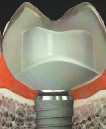
INDIVIDUELLES ZWEITEILIGES ABUTMENT (Klebebasis und ZrO 2 -Aufbau)
